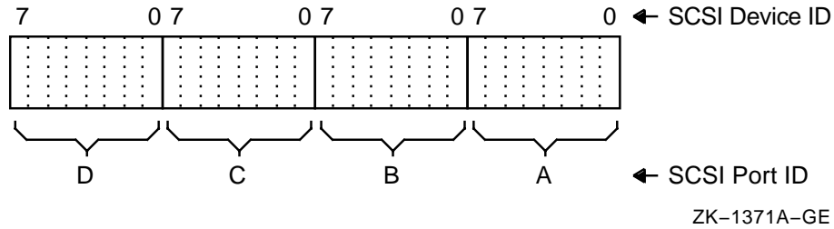
Figure 17–6 SCSI_NOAUTO System Parameter
